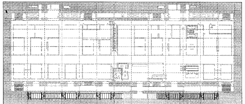
Mnam/Cci : les futurs espaces du niveau 4.
