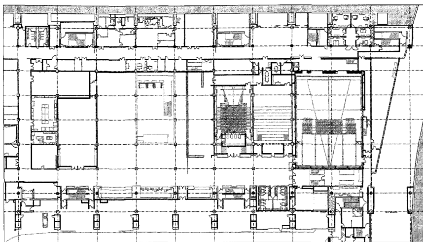
Les futurs espaces du Pôle spectacles, niveau -1. (Plans mis à jour fin décembre 1998)
